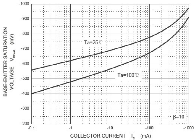
V_{BE} - I_c
