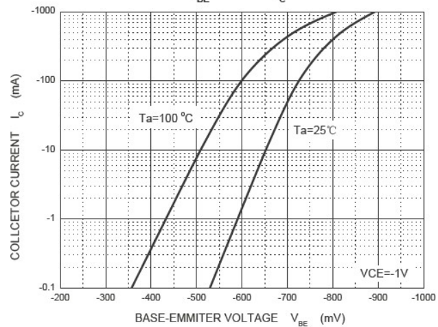
V_{BE} - I_c
